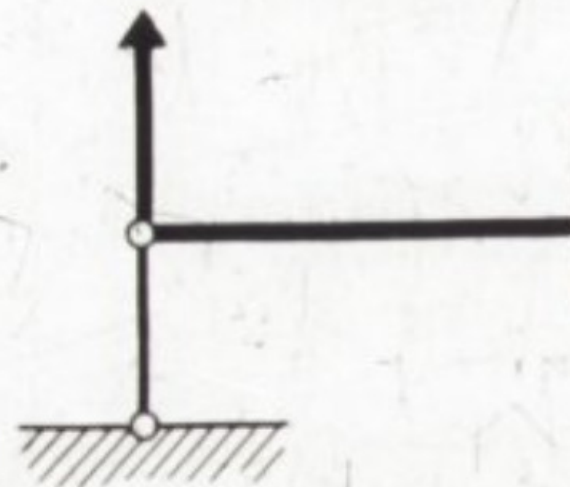
Расчетная схема
